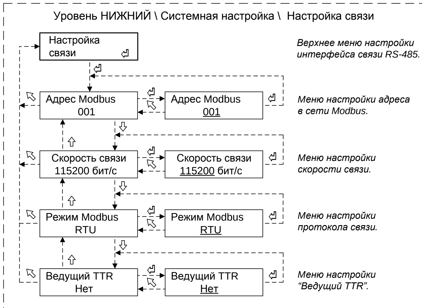
Рисунок 22 – Структура меню настройки сетевых параметров
