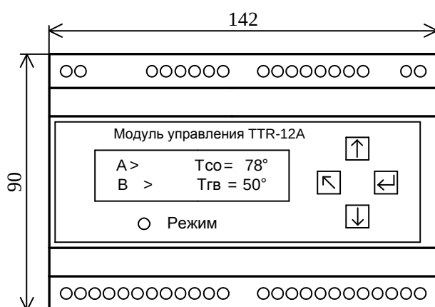
Рисунок Б.1 – Общий вид и габаритные размеры TTR-12A-230
