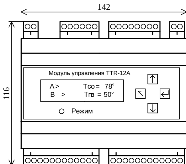
Рисунок Б.2 – Общий вид и габаритные размеры TTR-12AK-230
