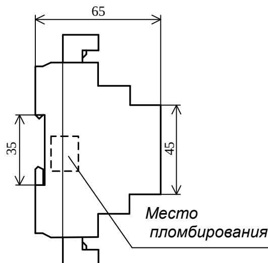
Рисунок Б.2 – Общий вид и габаритные размеры TTR-12AK-230
