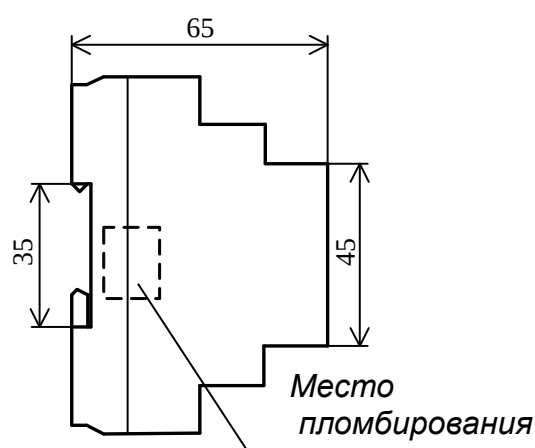
Рисунок Б.1 – Общий вид и габаритные размеры TTR-12A-230
