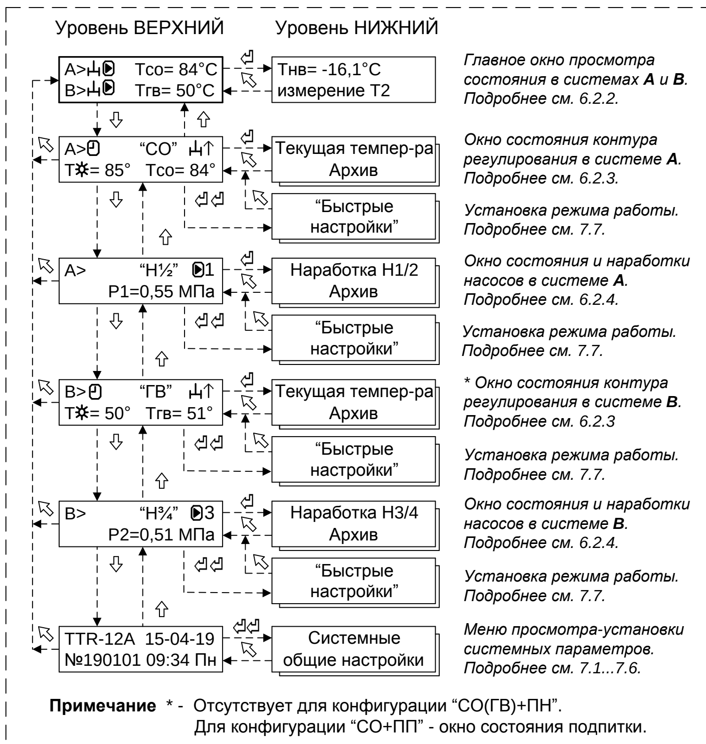
Рисунок 3 – Общая структура пользовательского меню
