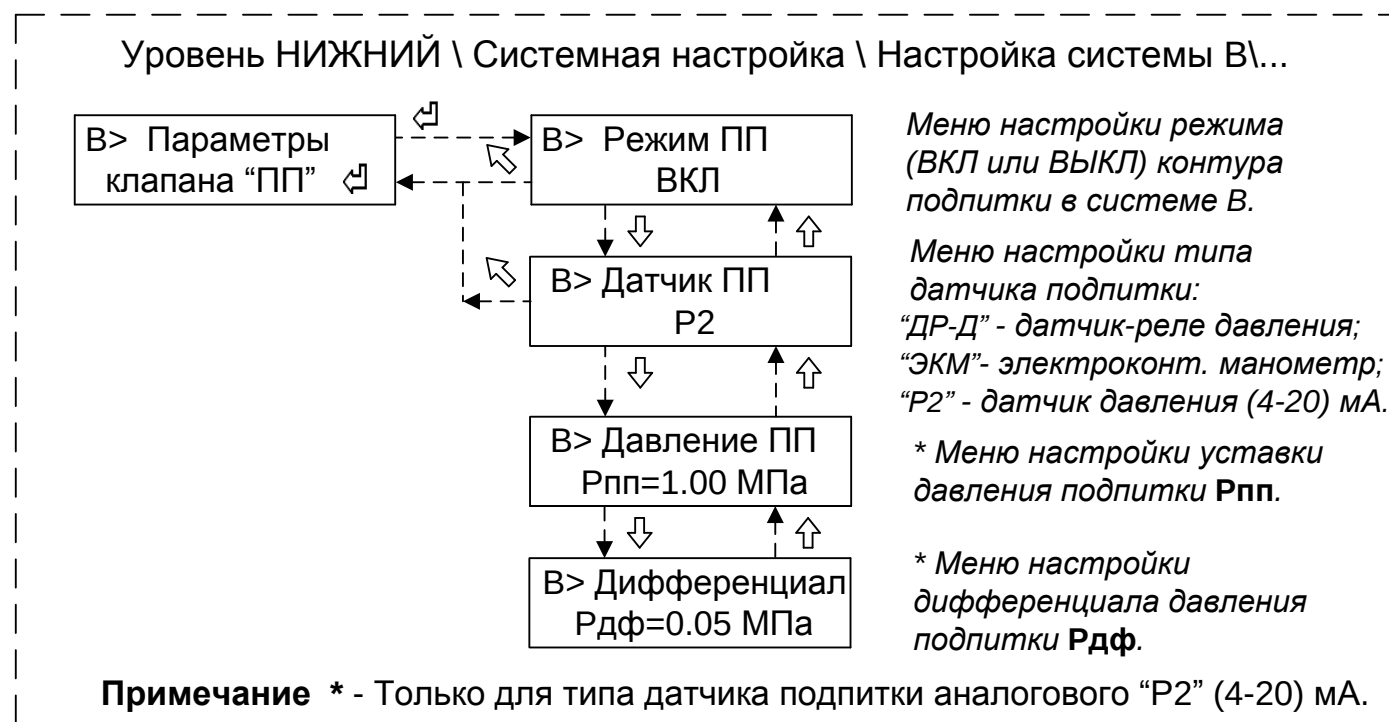
Рисунок 13 – Структура меню настройки параметров контура “ПП” (Подпитка)
