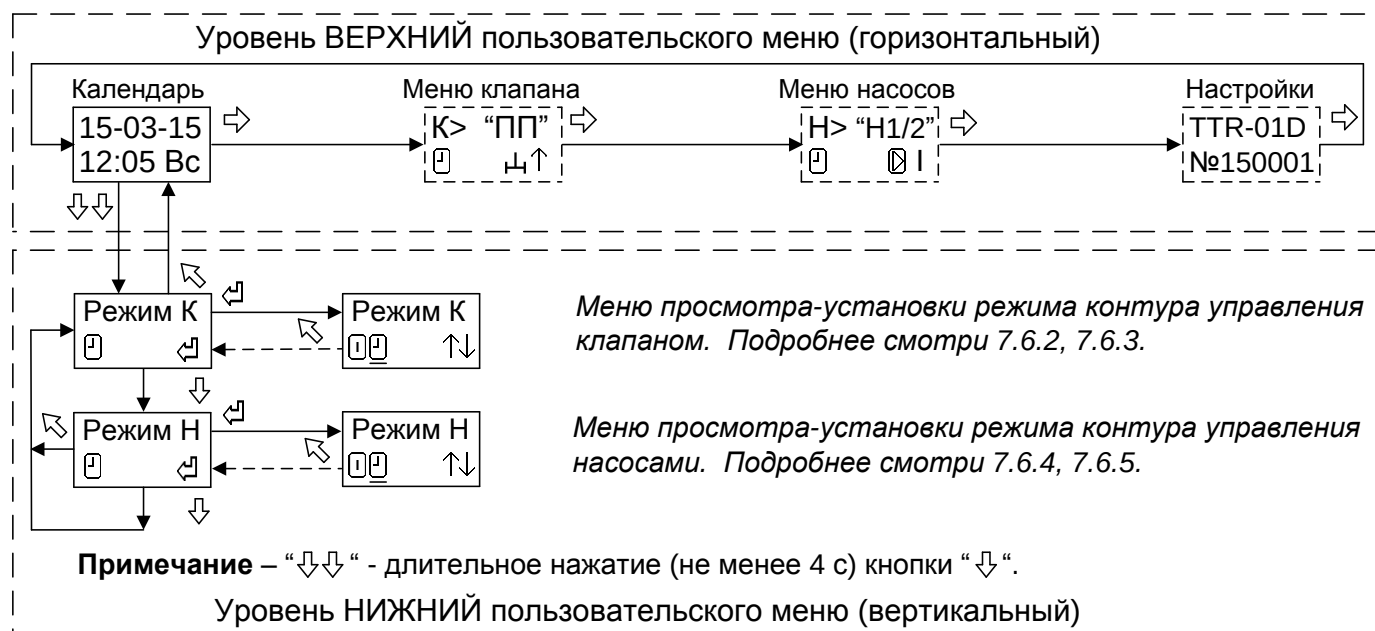
Рисунок 7 – Структура меню настройки режима работы контура
