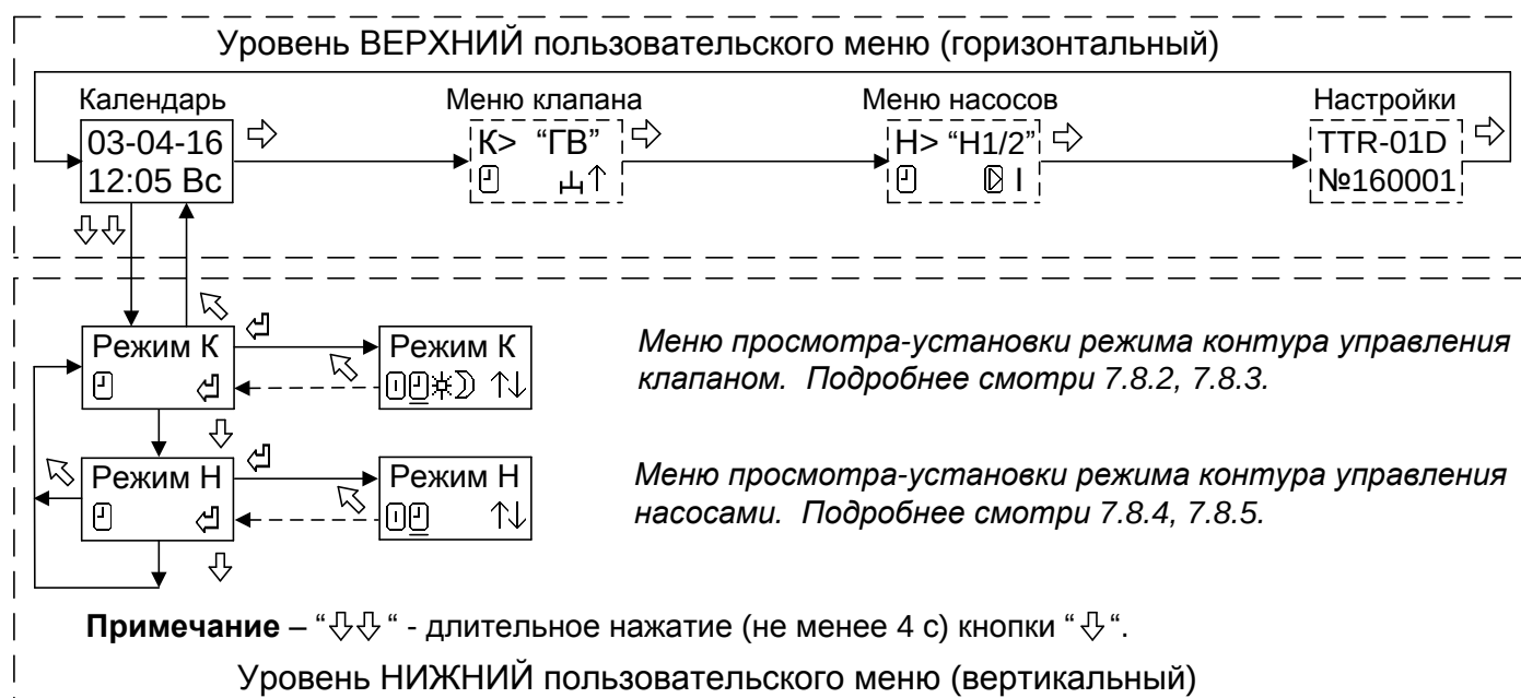
Рисунок 13 – Структура меню настройки режима работы контура
