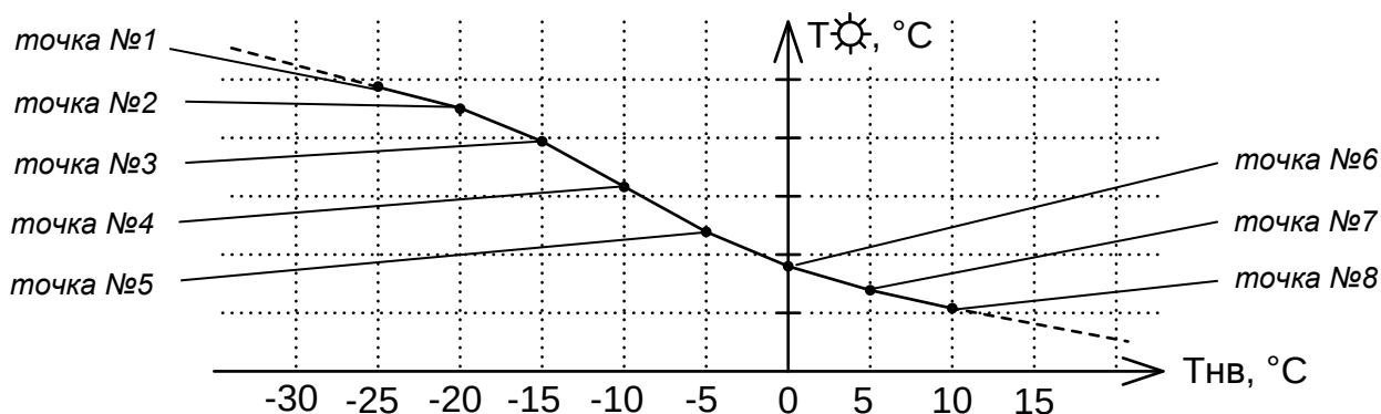
Рисунок 7 – Температурный график
