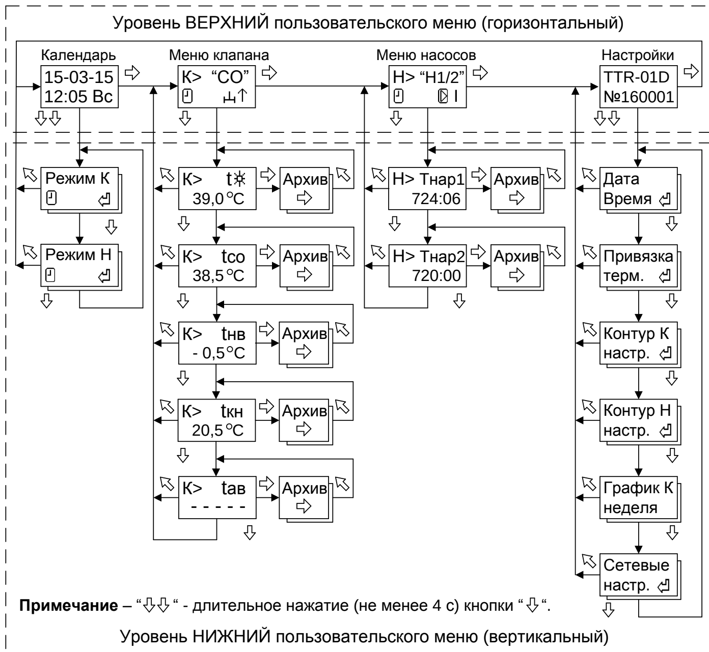
Рисунок 2 – Общая структура пользовательского меню
