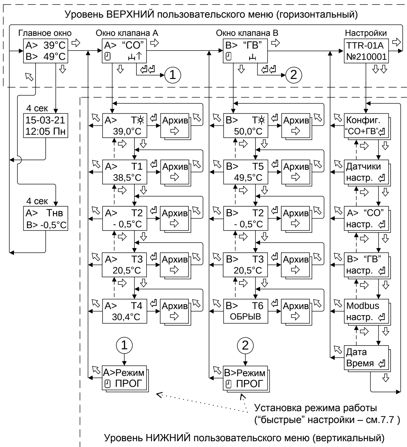
Рисунок 4 – Общая структура меню для конфигурации "2СО", "СО+ГВ", "2ГВ"
