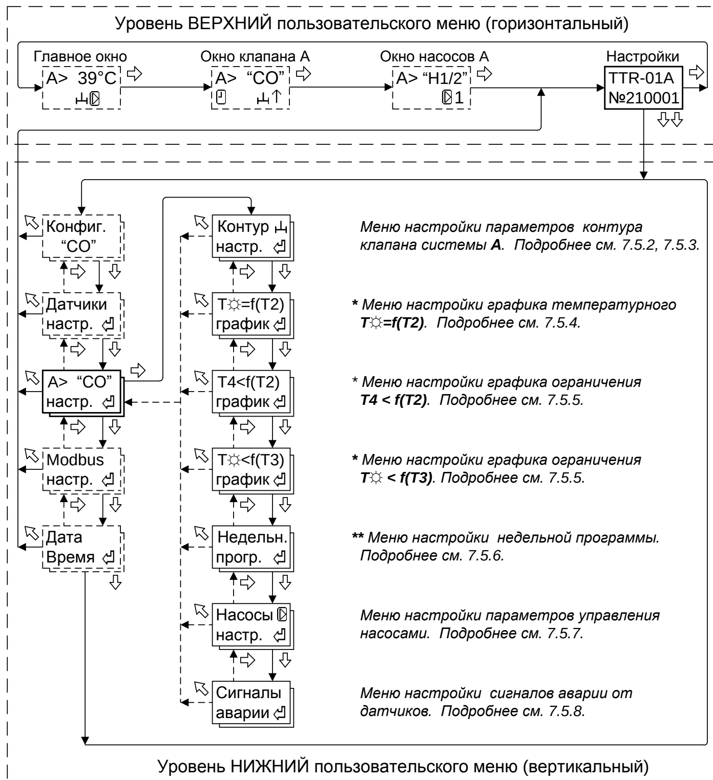
Рисунок 12 - Структура меню настройки параметров
