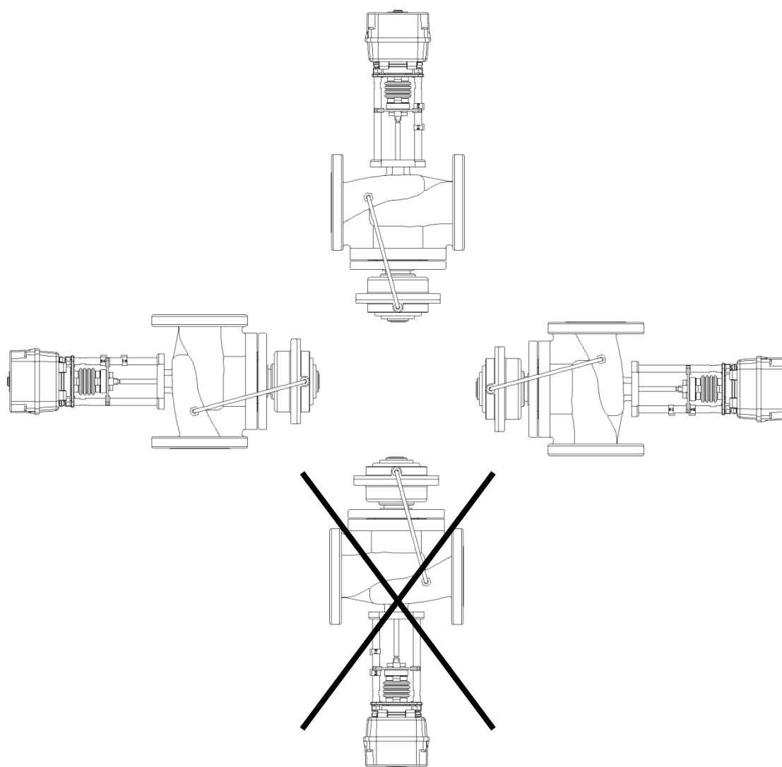
Рисунок А.2 Монтаж клапана.
