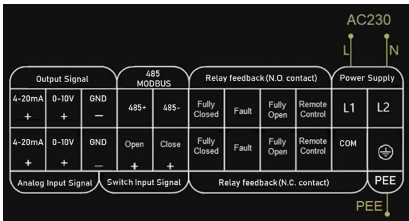
Рис.Б.1 Электрическая схема подключения переменного тока напряжением 230 В
