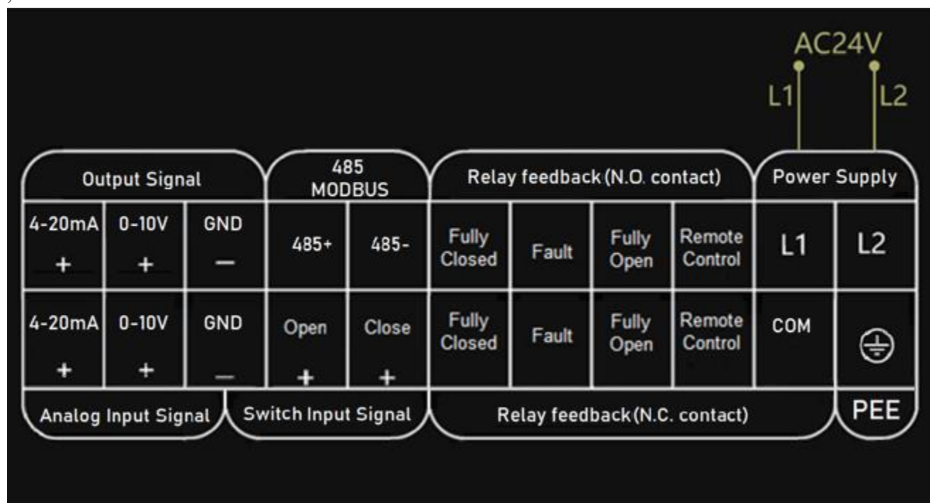
Рис.Б.2 Электрическая схема подключения переменного тока напряжением 24 В
