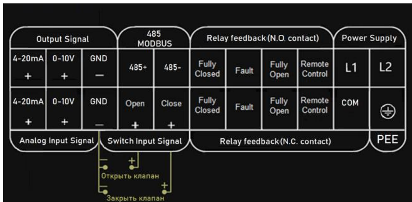
Рис. Б.6. Схема подключения 3-х позиционного управления (пассивный контакт)
