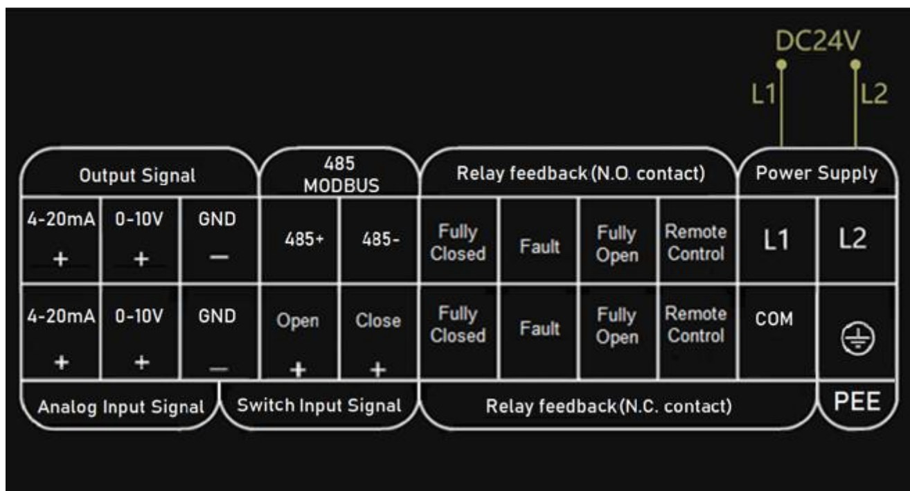
Рис.Б.3 Электрическая схема подключения постоянного тока напряжением 24 В
